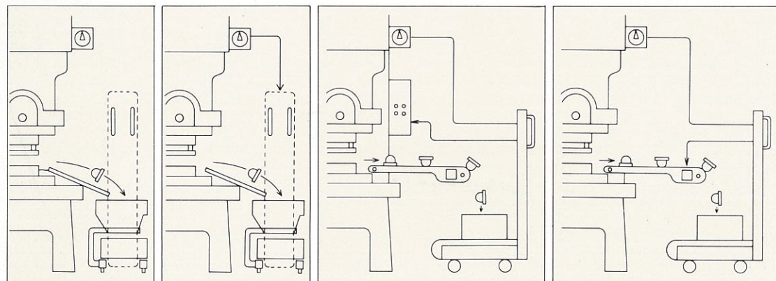
①センサ入力・シャッター連動 Sensor-shutter interlocking operation.
