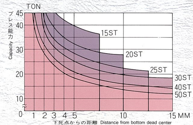
■トルク能力線図/ Torque capacity graph
