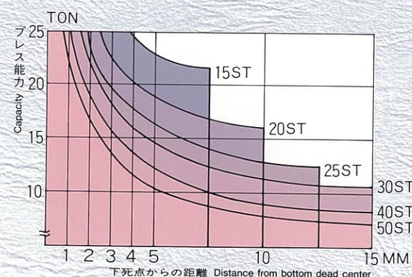
■トルク能力線図/ Torque capacity graph
